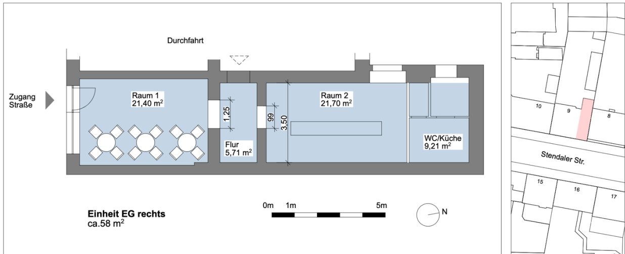
GRUNDRISS
